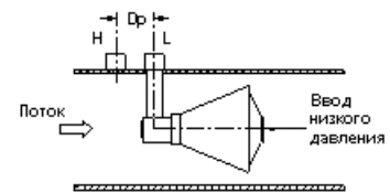
Вводы высокого и низкого давления Рисунок 16
