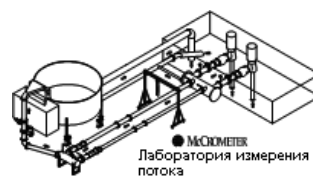
Калибровочная гравиметрическая 40 килофунтовая (181,44 кг-овая) установка
