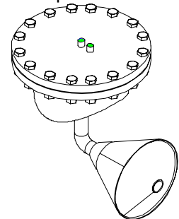
V-Cone de tapa superior de inserción Figura 9
