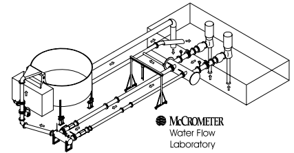
Inst. de calibr. 40k gravimétrico Figura 10
