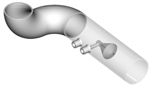
Dos codos y el V-Cone Figura 5
