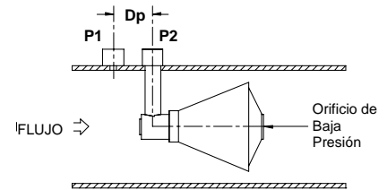
Orificios de alta y baja presión Figura 1
